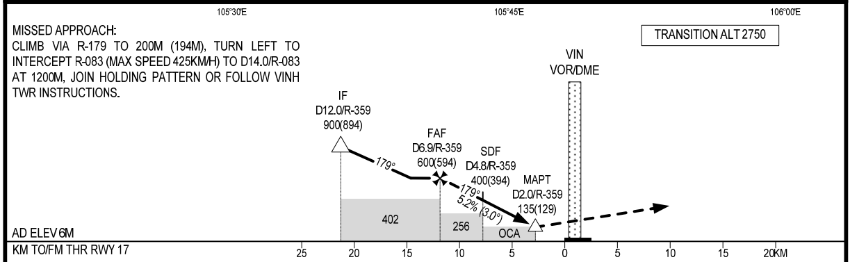
FAF - MAPT: 4.9NM (9.1KM)
